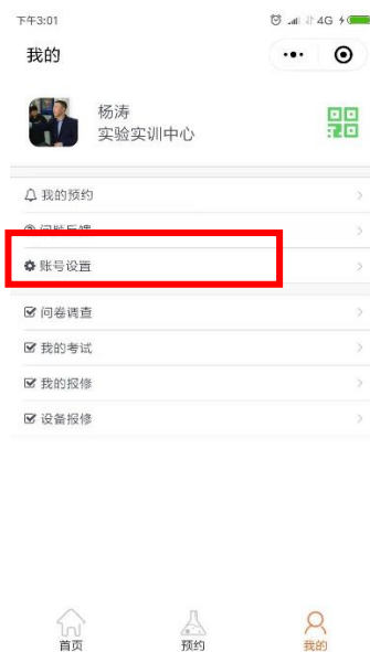
登录后界面
